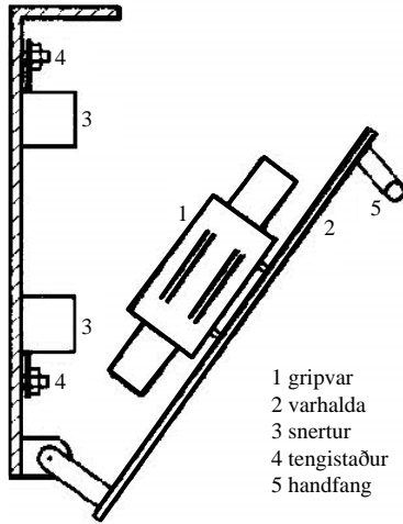
Einföld mynd af gripvarrofa.
