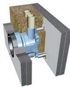
Apparát-dosa AU5.5
