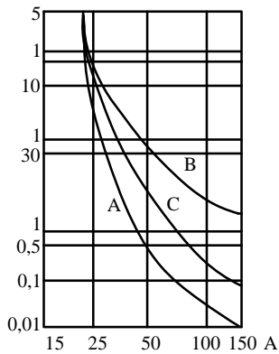
Kennilínur bræðivara.
