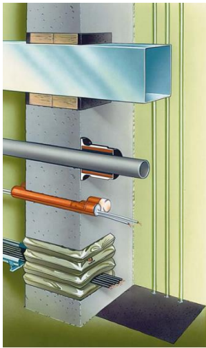
Brunaþétting með pípum og strengjum.
