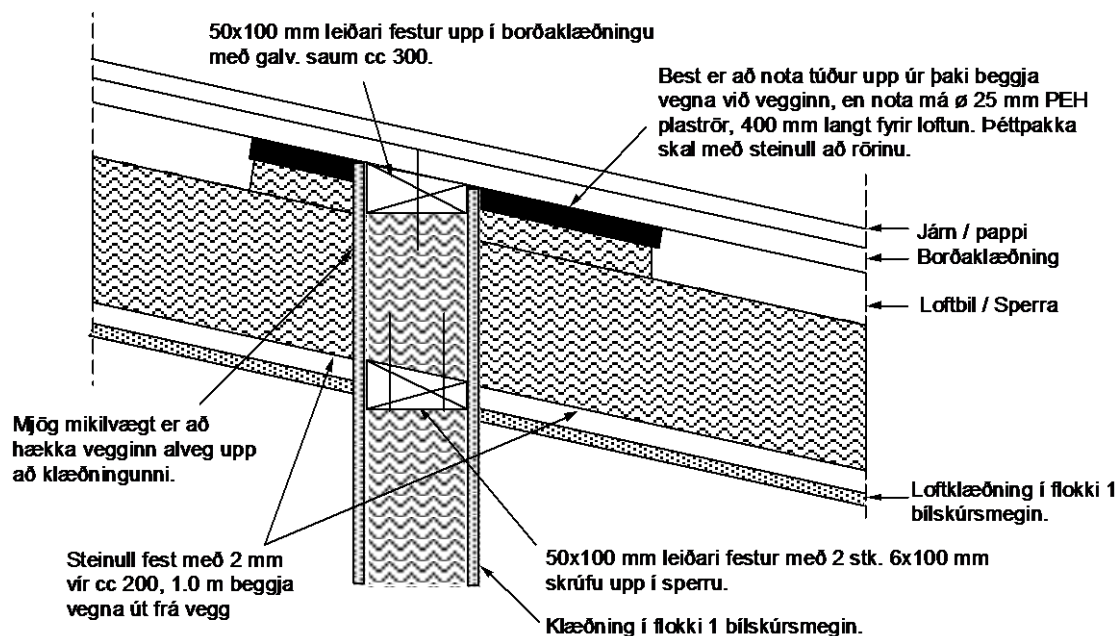
Mynd 5 Frágangur á Ei60 vegg við þak. Veggurinn liggur þvert á sperrur.
