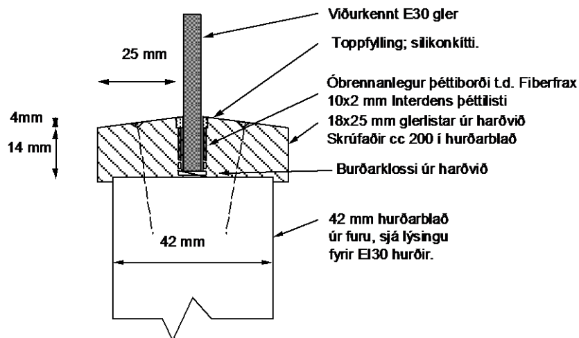
Mynd 15 Frágangur á E30 gleri í hurð.
