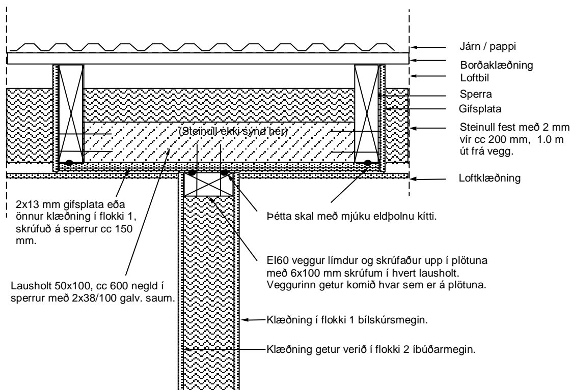
Mynd 4 Frágangur á Ei60 vegg við þak. Veggurinn kemur á lausholt og klæðningu á milli sperra.
